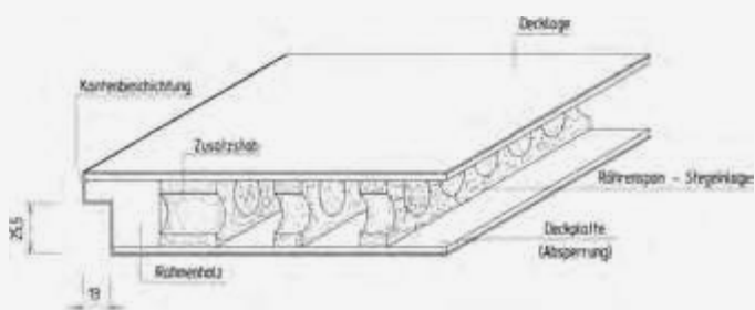
Innenleben einer Röhrenspanstreiftür
