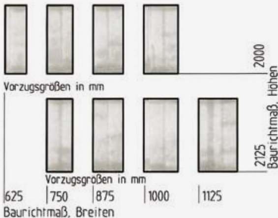
Rohbauöffnungen, die Vorzugsgrößen sind grau hinterlegt
