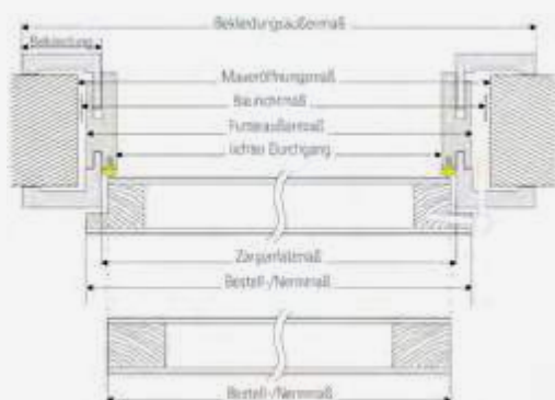
Zusammenfassung der relevanten Zargen/Türblattmaße
