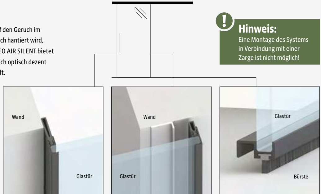
Eine Gummilippe dichtet direkt in die Wandleibung ab.
