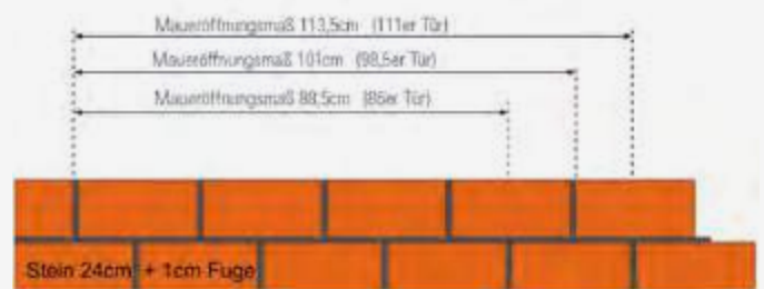
Baurichtmaße als Maßketten in der Breite
